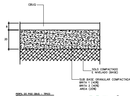
PERFIL DO PISO CBUQ – TÍPICO
